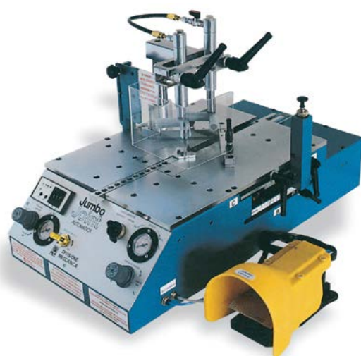
JUMBO JOINT AVTOMATIC - 2P, 3P Pnevmatski stroj za spajanje okvirjev z možnostjo dvojne ali trojne avtomatske nastavitve JUMBO JOINT AVTOMATIC - 2P, 3P Pneumatic frame assembling machine with the possibility of 2 or 3 automatic settings
